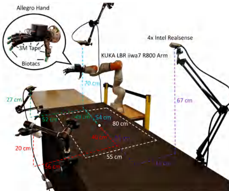
图6 DexPilot系统工作空间布局
